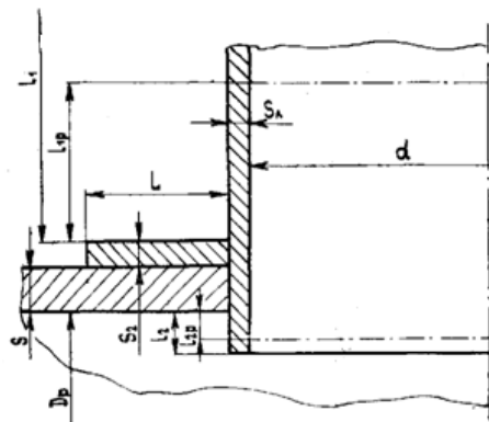
Рисунок 2 - Схема укрепления отверстия шуцером и накладным кольцом
