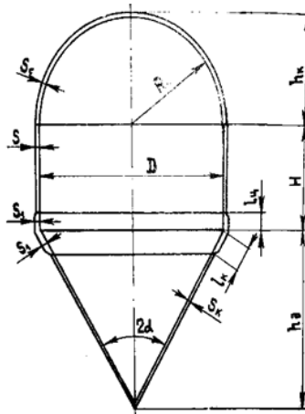
Рисунок 1- К расчету корпуса аппарата
